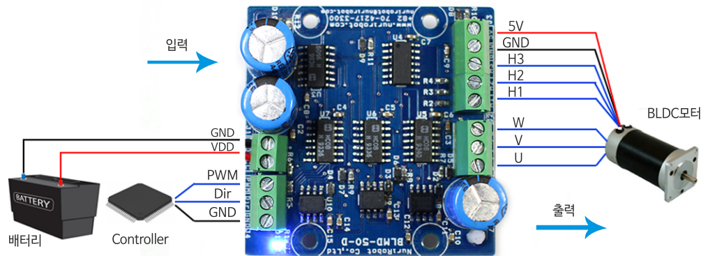
그림 2. BLMD-50-D 결선도
