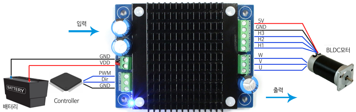
그림 2. BLMD-100-D 결선도
